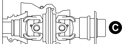
GIUNTO OMOCINETICO CONSTANT VELOCITY JOINT
