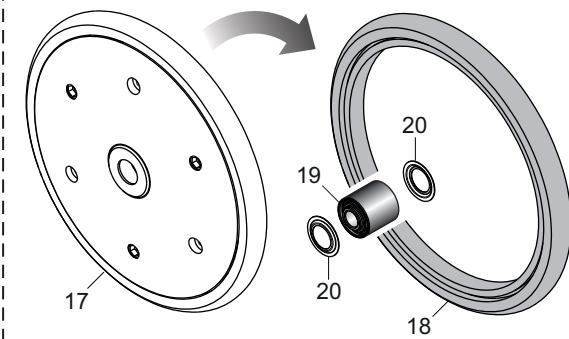
1" «V» SHAPED RUBBER PRESS WHEEL
