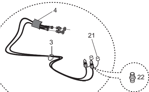
KIT RIDUZIONE TUBI IDRAULICI OPTIONAL OPTIONAL HYDRAULIC TUBE REDUCTION KIT
