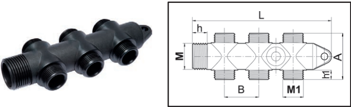
Raccordo collettore a 3-6 vie 3-6 way fitting Colector roscado de 3-6 vías
