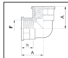
Raccordo filettato curvo 90° femmina/femmina 90° female/female fittings Racor curvo 90° hembra/hembra
