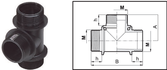
Raccordo filettato a "T" maschio Male Tees fittings Racor en "T" macho
