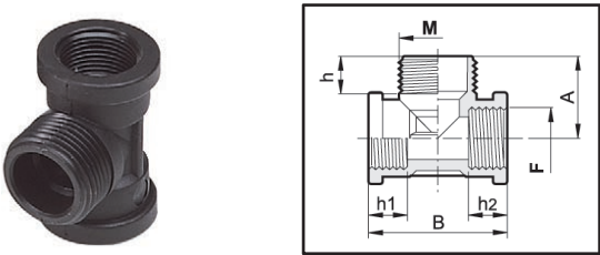
Raccordo filettato a "T" maschio/femmina Male/female Tees Racor en "T" macho/hembra
