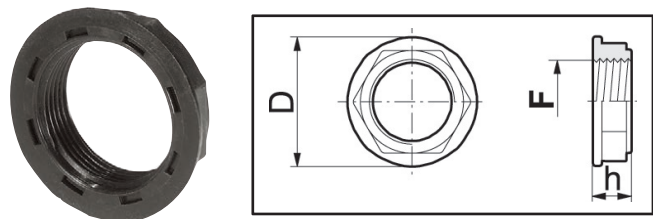
Ghiera Lock ring Tuerca
