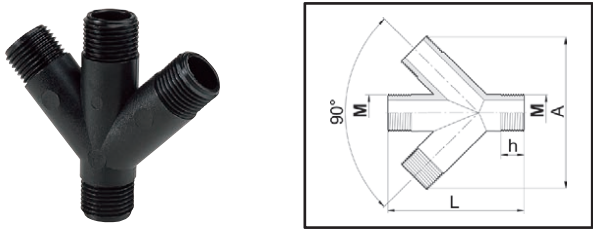
Raccordo filettato a 4 vie 45° maschio 45°, four-way male fitting Racor de cuatro vías a 45° macho
