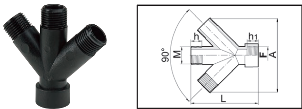
Raccordo filettato a 4 vie 45° maschio/femmina 45°, four-way male/female fitting Racor de cuatro vías a 45° macho/hembra
