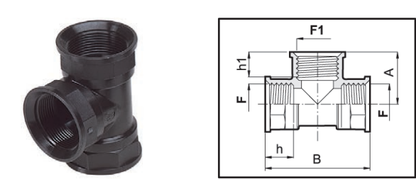
Raccordo filettato a "T" femmina Female Tees fittings Racor en "T" hembra
