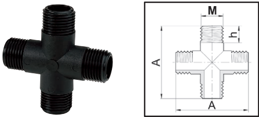
Raccordo filettato a 4 vie 90° maschio 90°, four-way male fitting Racor de cuatro vías a 90° macho
