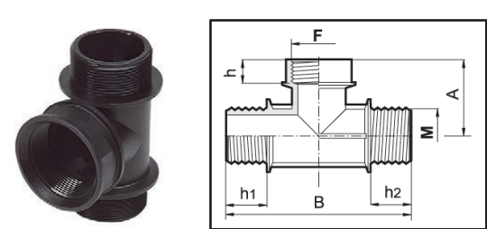
Raccordo filettato a "T" femmina/maschio Female/male Tees fittings Racor en "T" hembra/macho
