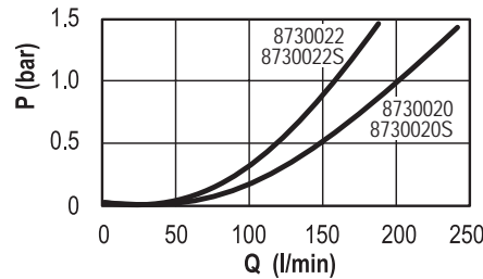
Caduta di pressione con valvola tutta aperta Pressure drop with fully open valve Caída de presión con válvula toda abierta
