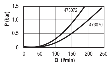
Caduta di pressione con valvola tutta aperta Full open valve pressure drop Perdita de caudal a válvula abierta
